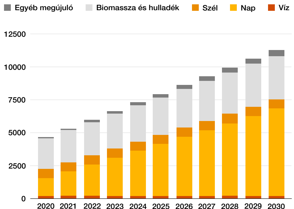
Villamosenergiatermelési-kapacitás felfutása (MW)
